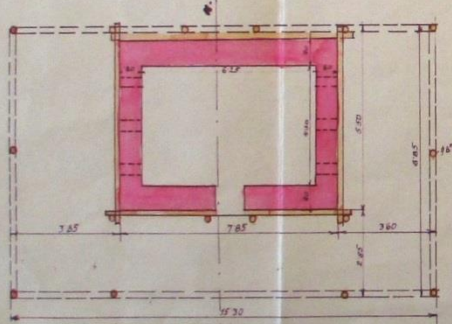
Talliskiviabi, põhiplaan 1:100
